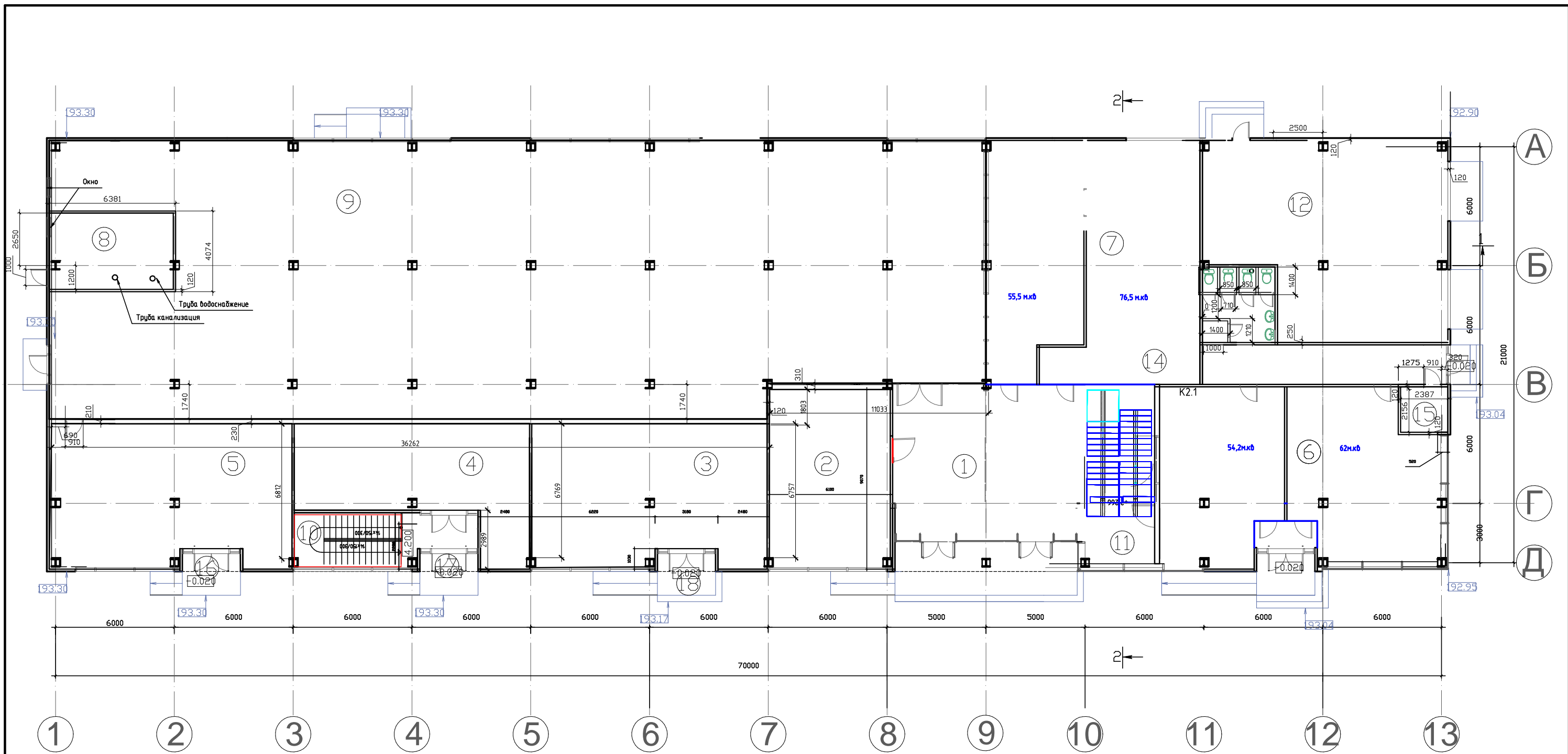
Экспликация помещений 1 этажа
